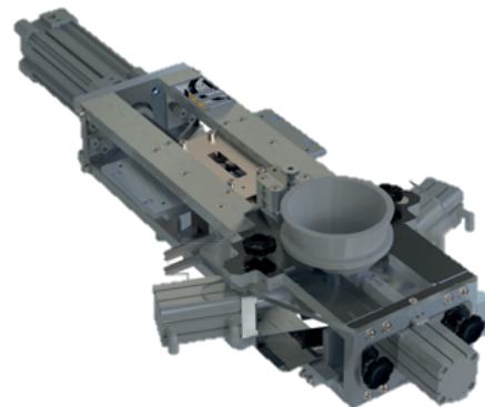
Устройство формирования клипсы (клипсатор)
